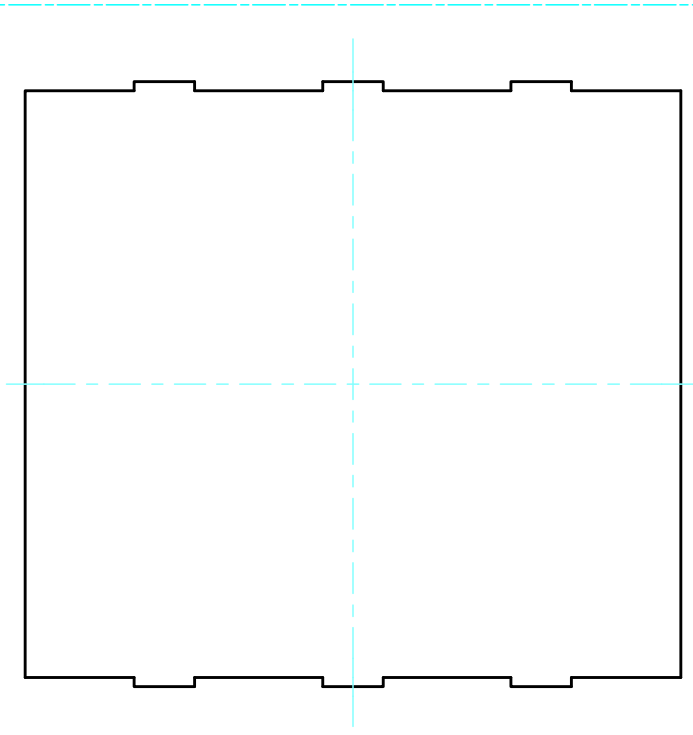
Dパネル2裏面 / D Panel 2 Backside
